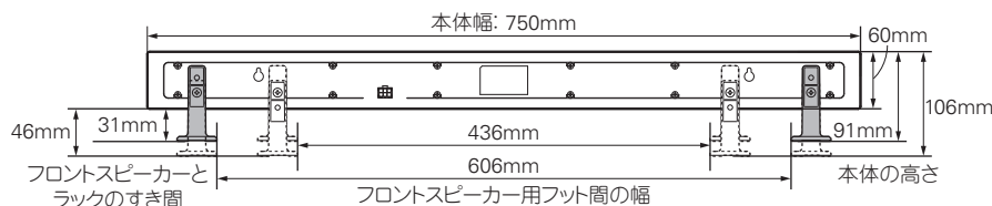
フロントスピーカー用フットの取り付け寸法図
