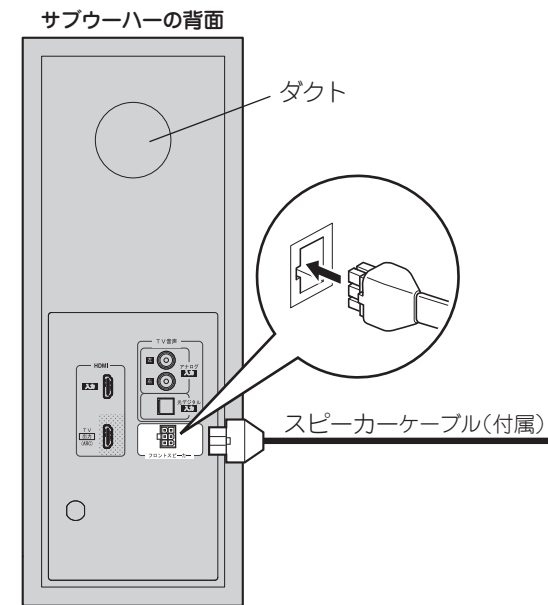
サブウーハーの背面
